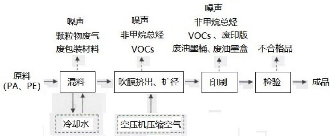
图 2-2 工艺流程及产物环节示意图
